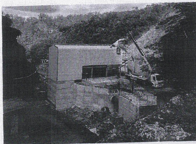
Fotos 1, 2 e 3 – demonstram a execução da estrutura metálica de fechamento da casa de força
