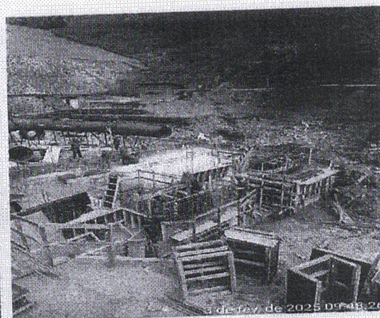
Fotos 3 demonstram a execução da estrutura de concreto para construção da casa de força
