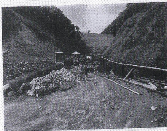
Fotos 3 demonstram a execução da estrutura de concreto para construção da casa de força
